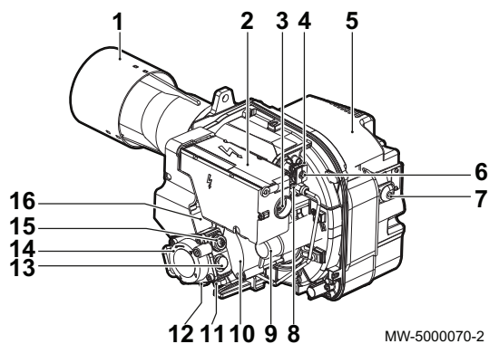
Fig.3 Principaux composants
